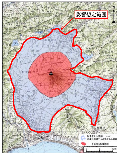
図2 融雪型火山泥流の影響想定範囲
